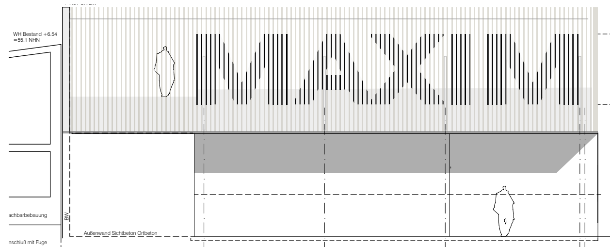
Gesamtansicht der Nordfassade M.1:125
